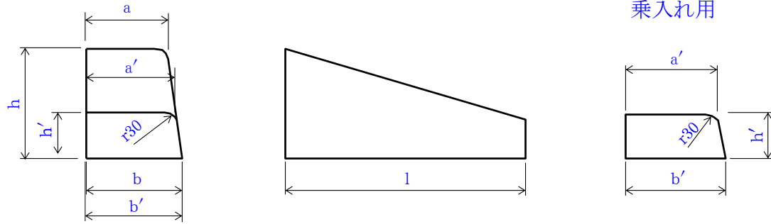
片面歩車道境界ブロック片下り
